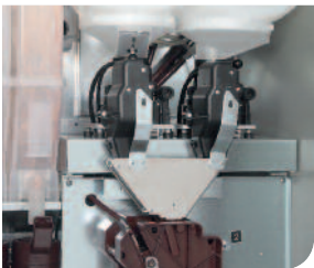
Due tipi di caffè con macinatura e dosatura indipendenti
